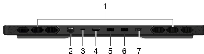
Figure 5. Legion Pro 7 16IRX9H—vue arrière
