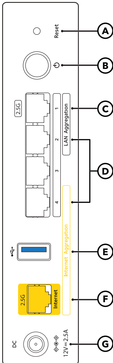
Illustration 3 : Panneau arrière
