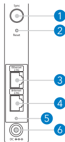
Routeur Orbi
