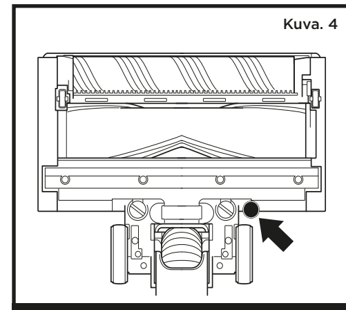
FLOORDETECT- LATTIANTUNNISTUSANTURI
