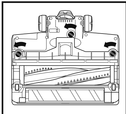
ANTI-HAIR WRAP-BODENDÜSE
