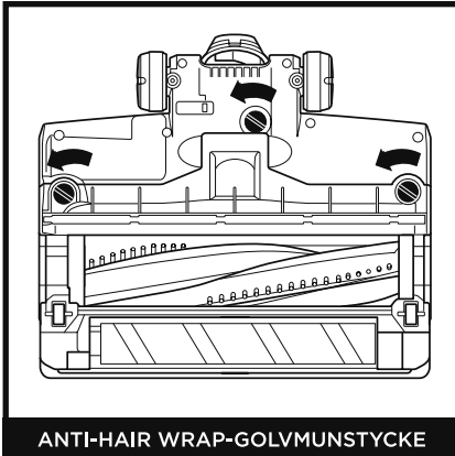
ANTI-HAIR WRAP-GOLVMUNSTYCKE
