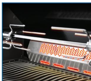
Brûleur infrarouge arrière pour des plats croustillants préparés avec une rôtiroisire
