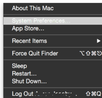
Рисунок 1. Меню Apple.
