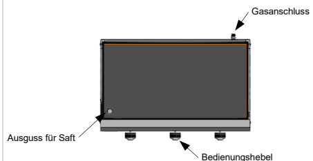
Beschreibung der Draufsicht des Plancha-Geräts
