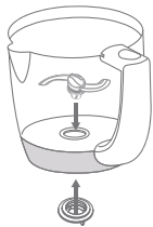
Αποσυναρμολόγηση
