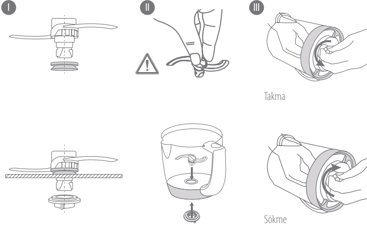
Sökme
