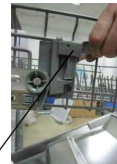
Languette pour le réglage en hauteur
