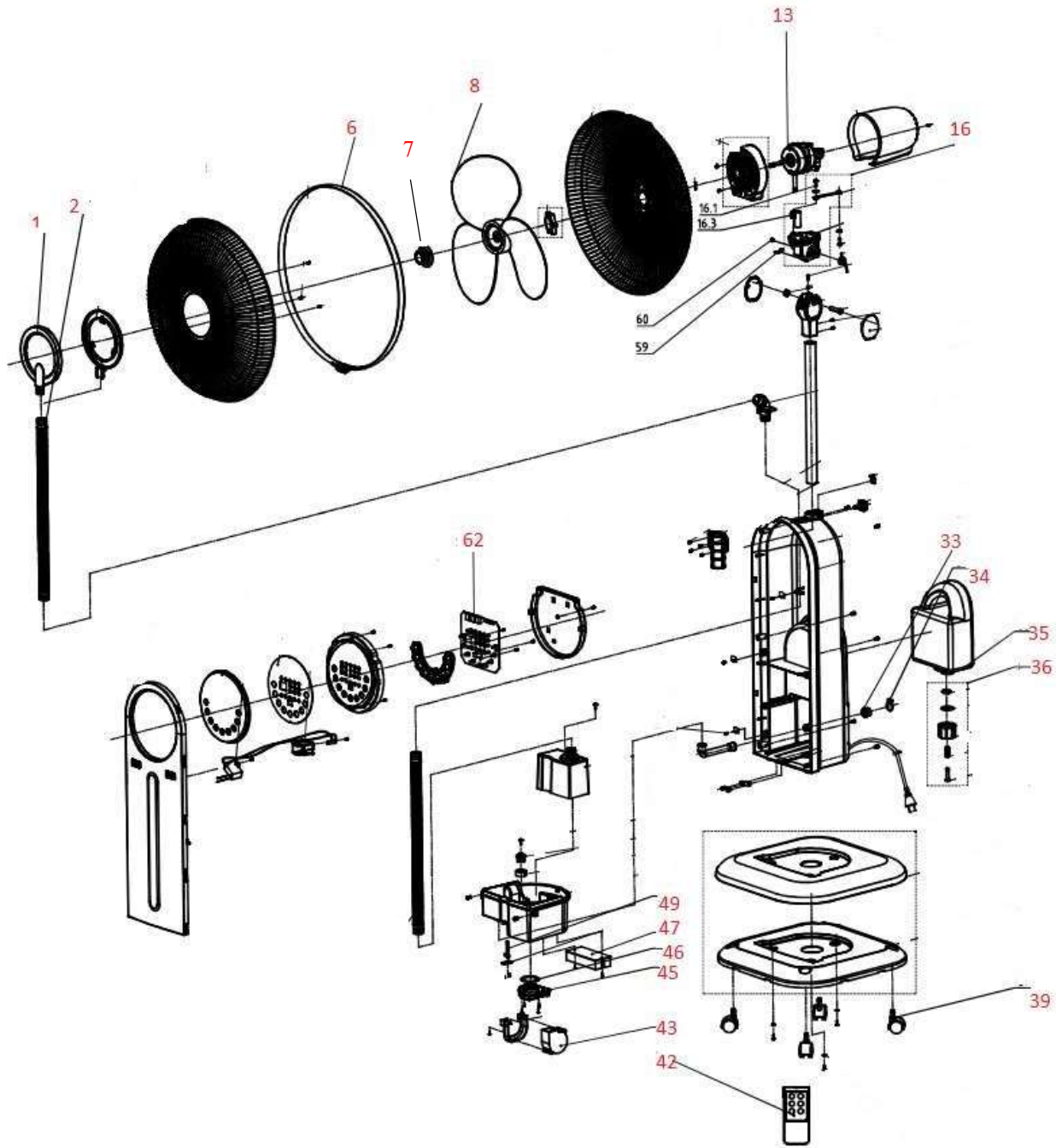
EVB2240N_ 8007889 Vue éclatée / Exploded view
