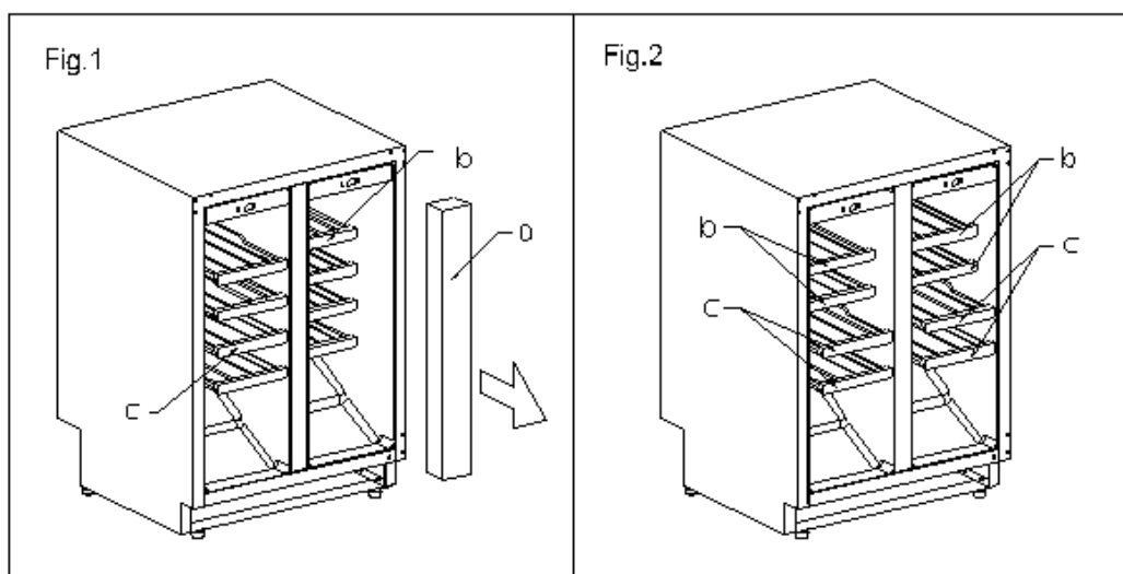
a. kartonnen doos met reserveonderdelen
