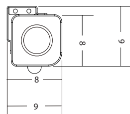
Côté du carter avec patte de fixation
