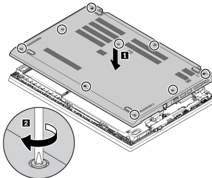
Figure 7. Installation du cache de la base pour les ordinateurs ThinkPad L580
