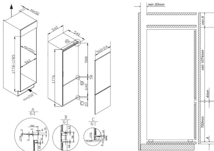
Schéma d'encastrement :
