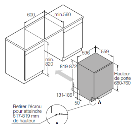
Dimensions d'encastrement
