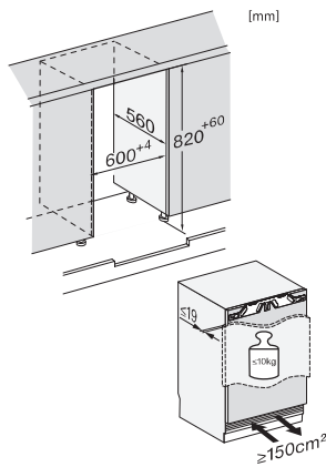
KU7016D, KU7015D, KU7035D, FNUS7040D, Built-under, Einbauskeizze, Nischenmaß (installation drawings)
