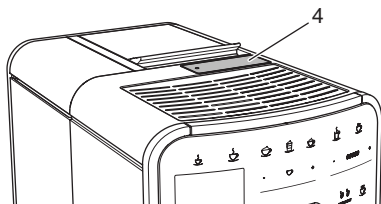
图 10: 咖啡粉斜槽
