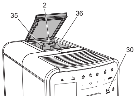
그림. 8: BARISTA TS의 2칸식 원두 용기
