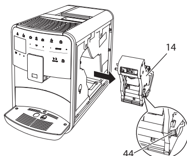
Afb. 21: Zetgroep demonteren, 2
