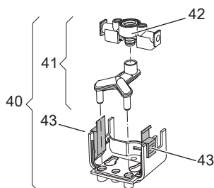
图 24: 拆卸出奶装置，图2
