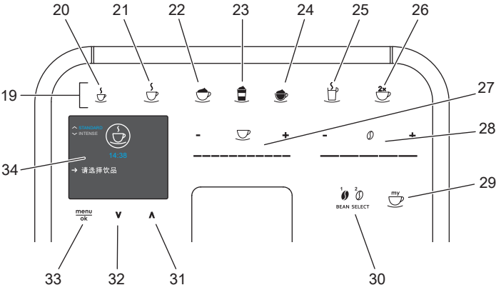
图 3: 操作面板
