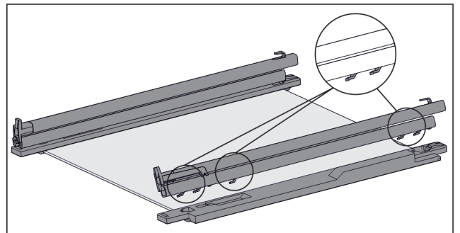
Fig. 34 Tablette en verre avec rails et pièces de retenue
