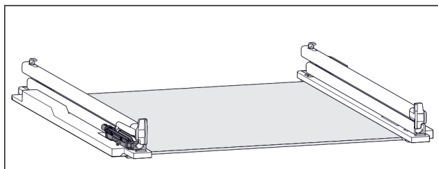
Fig. 37 Unité d'amortissement
