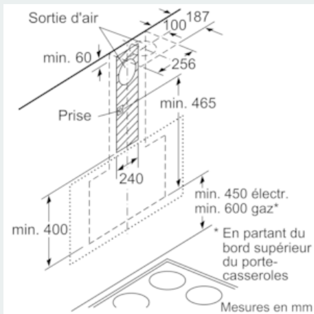
(1) Emplacement de la prise Respecter l'épaisseur maximale de la paroi arrière. Mesures en mm
