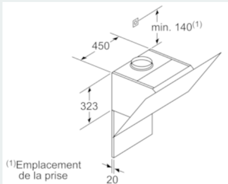
Appareil en mode circulation d'air sans canal set circulation d'air requis Mesures en mm
