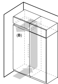
B: Sortie d'air \geq 600 \text{ cm}^2
