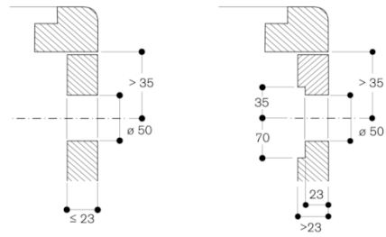
Installation du bouton de commande, encastré affleurant
