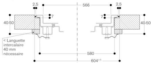
Coupe transversale
