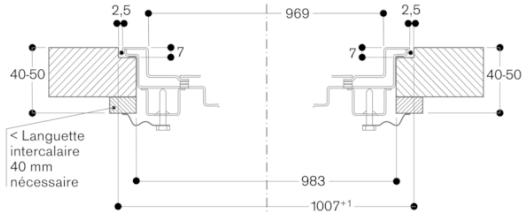
Coupe longitudinale
