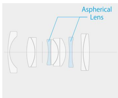
Schéma optique
