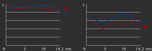
A 200mm Fréquence spatiale 15 l/mm et 45 l/mm
