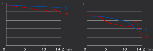
A 200mm Fréquence spatiale 15 l/mm et 45 l/mm
