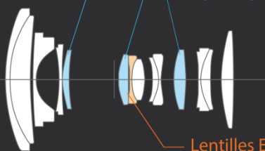
Lentilles asphériques
