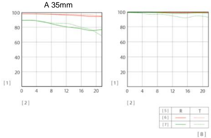
Courbes MTF : fréquence spatiale
