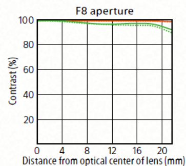
Courbes MTF : fréquence spatiale
