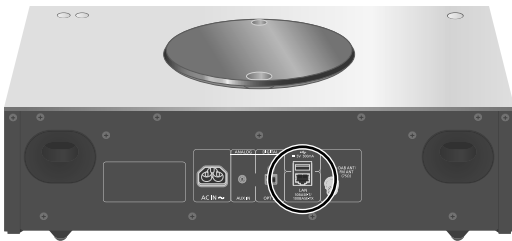
Câble réseau (LAN) (non fourni)
