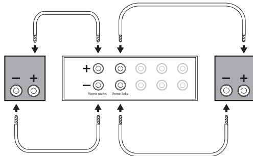
ABBILDUNG 3 STANDARDANSCHLÜSSE
