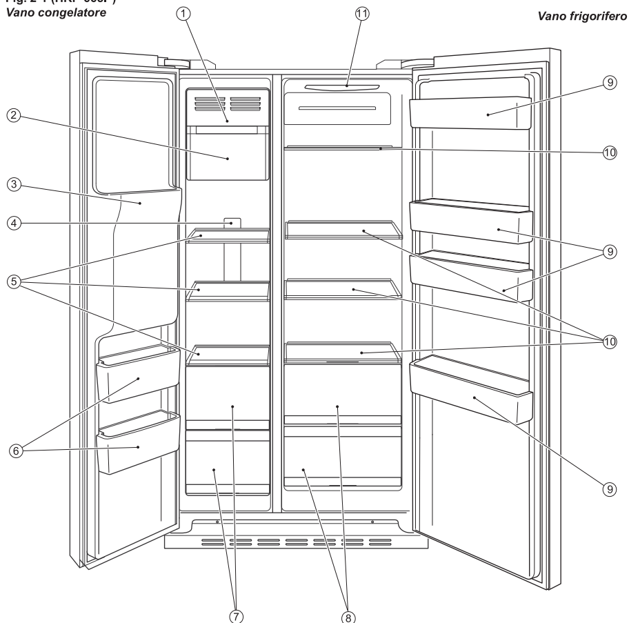
Fig. 2-1 (HRF-665I*) Vano congelatore
