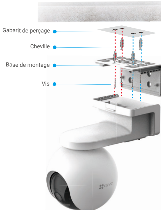
Fig. 1 Montage au plafond
