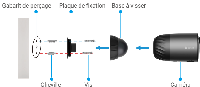
Fig. 1 Fixation par base vissée
