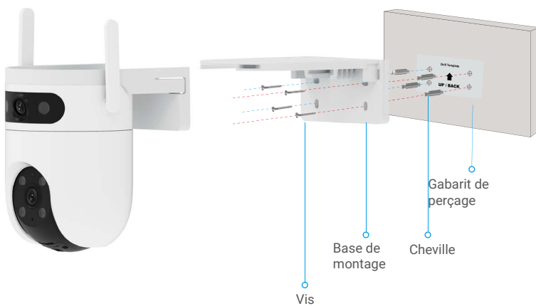
Fig. 2 Montage mural
