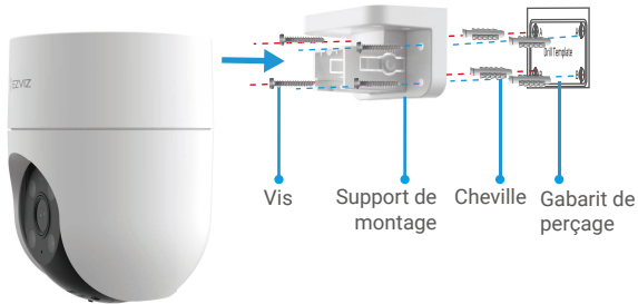
Fig. 2 Montage mural
