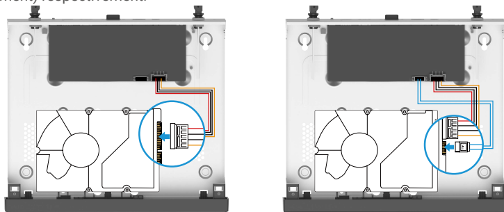
Connexion de câble de données
