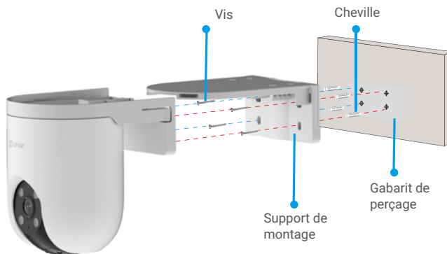
Fig. 2 Montage mural
