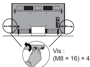
Figure 2 Tournez dans le sens antihoraire pour retirer
