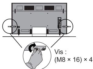
Figure 1 Tournez dans le sens horaire pour fixer
