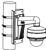
DS-1275ZJ-SUS Montage sur poteau vertical
