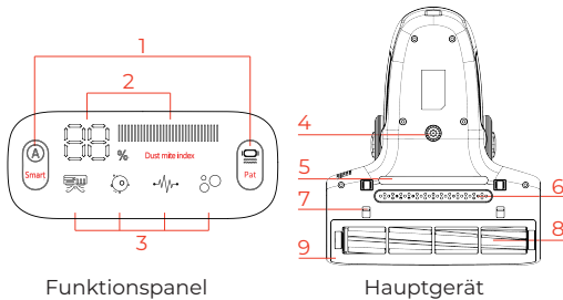
Funktionspanel
