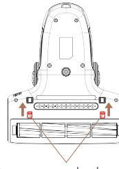
Deux serrures de plaque de fond
