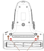
Zwei Bodenplattenschlösser
