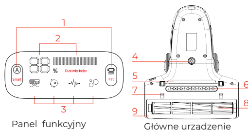
Główne urządzenie
