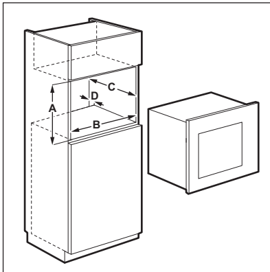
Distances d'installation
