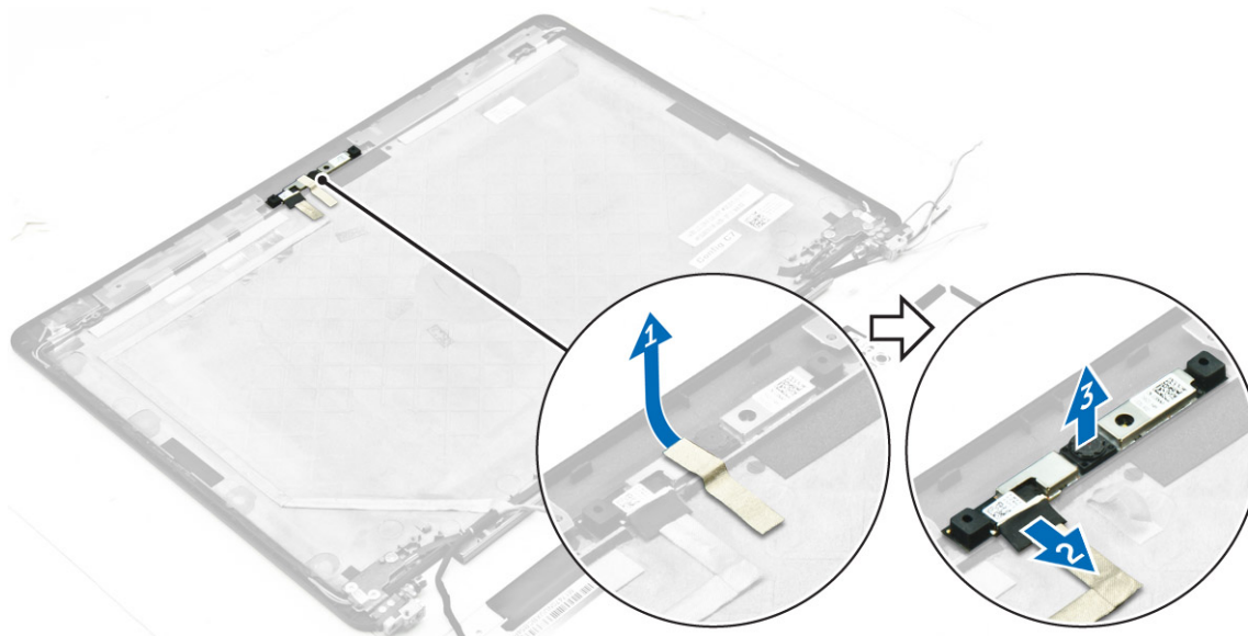
Figure 5. Retrait de la caméra d'un système non tactile
