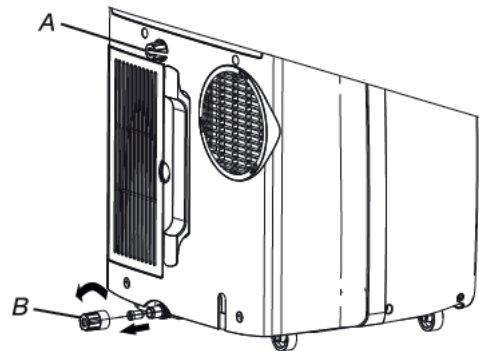
A. Горна тапа B. Маркуч за източване на кондензираната вода
