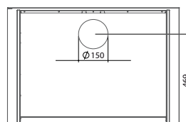
Emplacement de l'évacuation pour extraction horizontale
