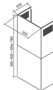
Cheminée en option
