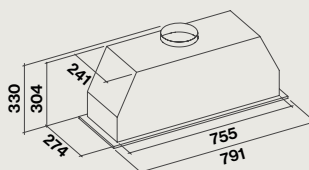
Dimension d'encastrement 762 mm x 245 mm
