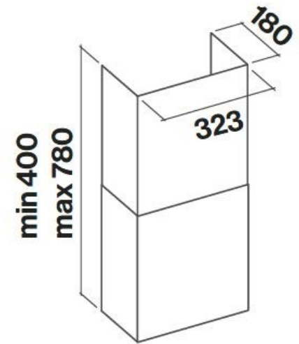
Optional chimney
