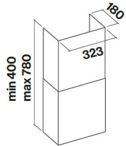
Optional chimney
