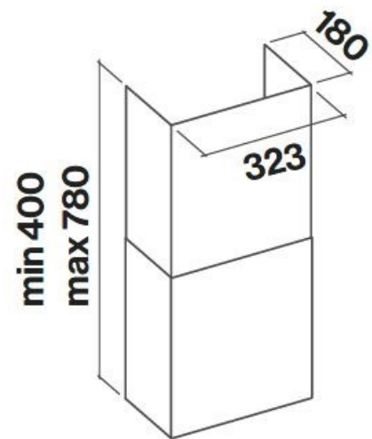
Optional chimney
