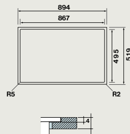
Installation à fleur Schéma d'encastrement
