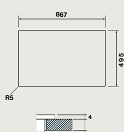
Installation semi-affleurante Schéma d'encastrement
