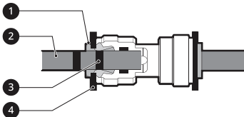
1 Douille de serrage 2 Tuyau 3 Insérer la conduite 4 Clip
